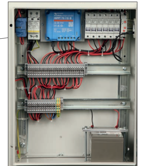
Coffret batterie + régulateur de charge.
