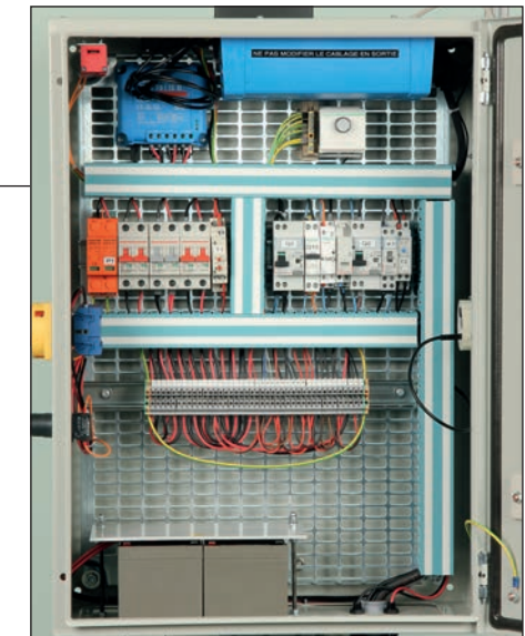
Coffret batterie + régulateur de charge.
