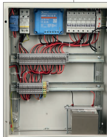
Coffret batterie + régulateur de charge.
