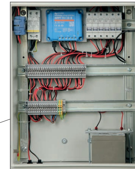
Coffret batterie + régulateur de charge.
