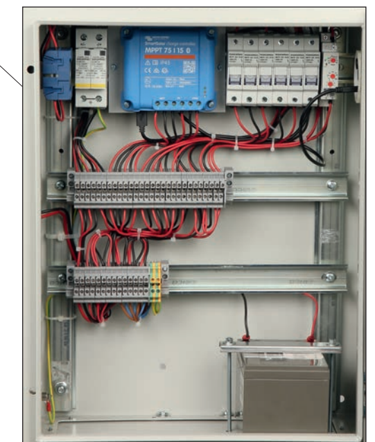
Coffret batterie + régulateur de charge. Bluetooth.
