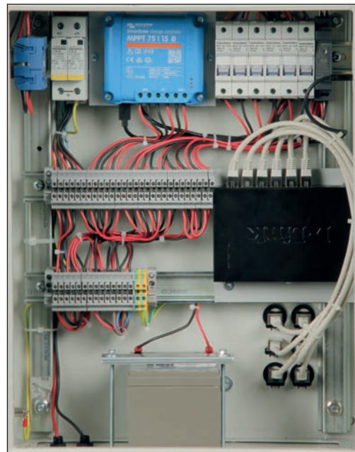
Vue intérieure de l'armoire électrique
