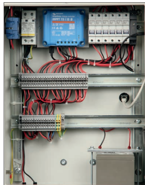
Coffret batterie + régulateur de charge. Bluetooth.
